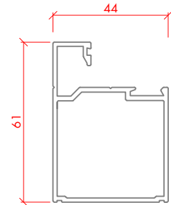
DOOR PILLAR POST PSL 315
